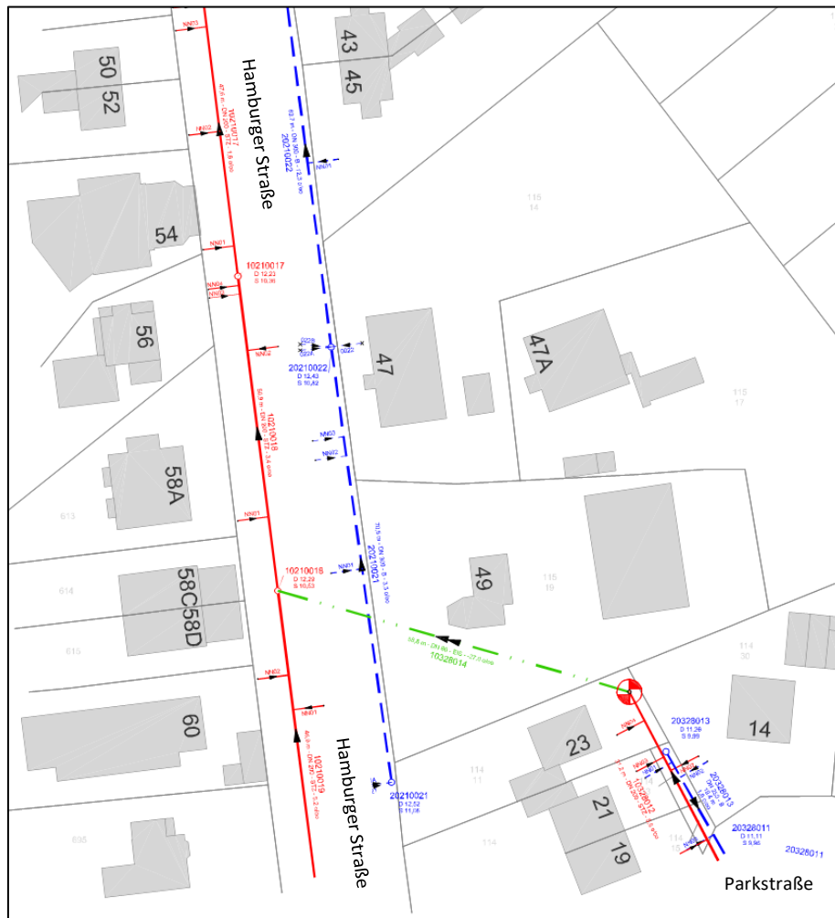
Abb. 1.6: Auszug aus dem Kanalkataster
